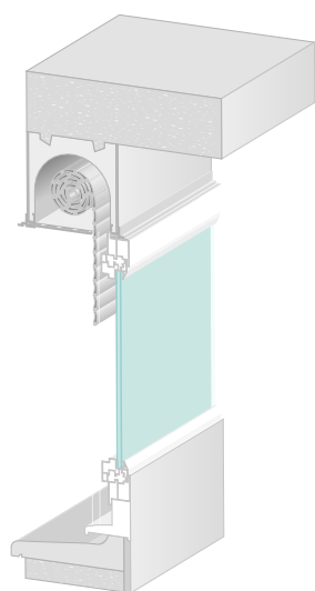
Enroulement extérieur
