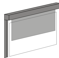
Guidage par coulisses zipées
